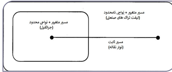
شکل ۲-۵. مشخصات مسیر و نواحی تجهیزات حمل و نقل
