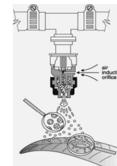
شکل ۱۹- نازل های القاء کننده هوا
