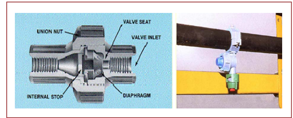
شکل ۱۴- شیرهای یک طرفه دیافراگمی
