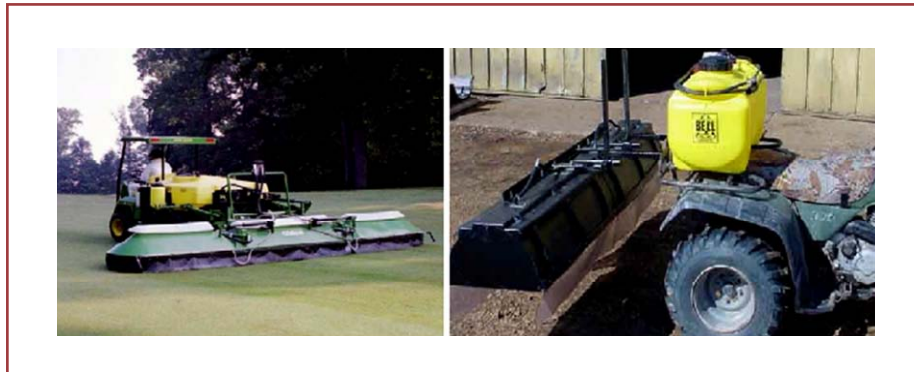
شکل ۲۰- سرپوش دار کردن سم پاش ها
