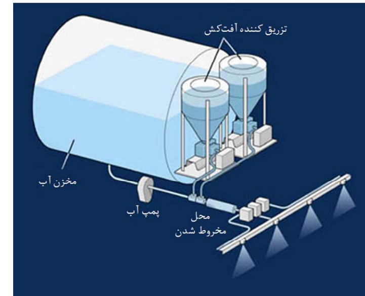
شکل ۱۱- سیستم تزریق مستقیم آفت کش
